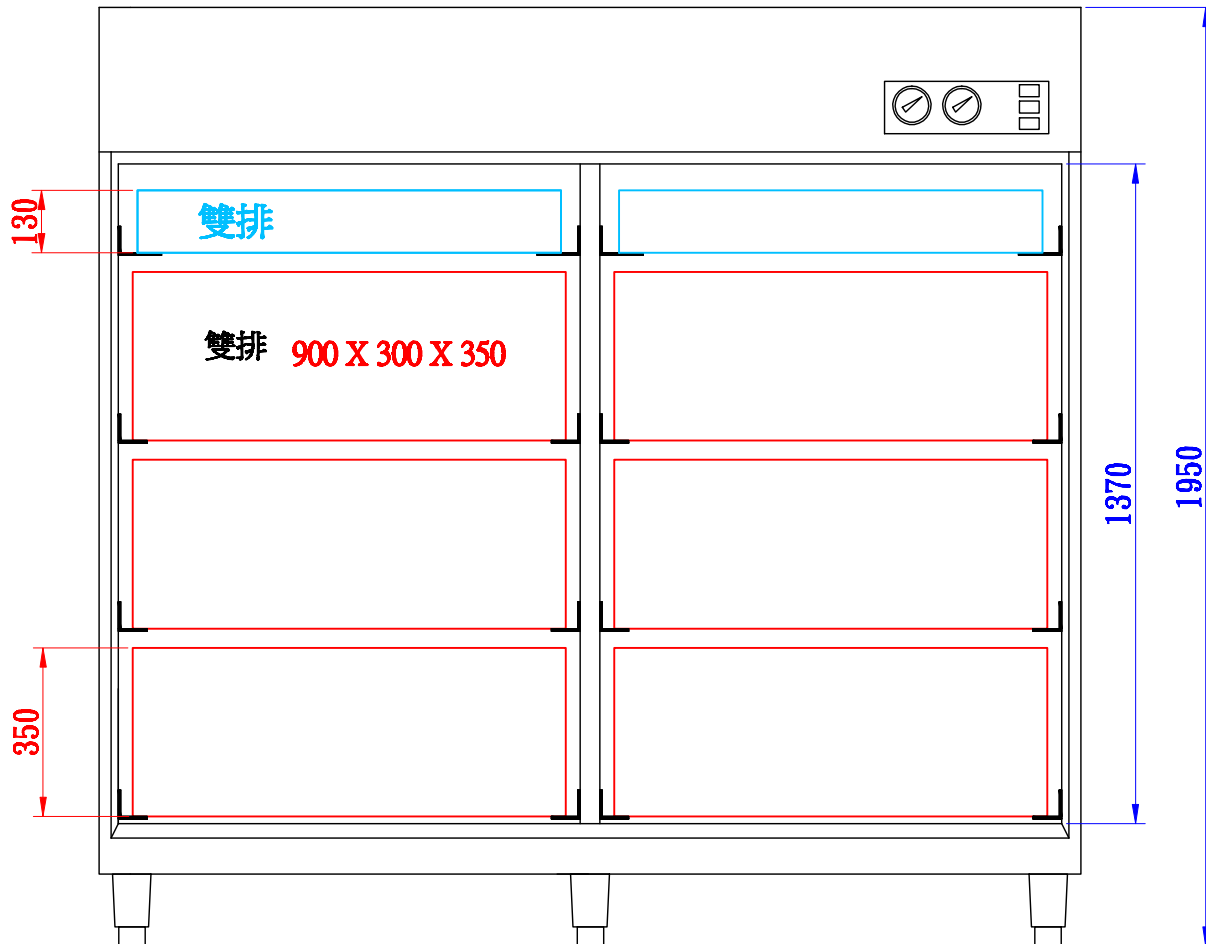
前視圖
