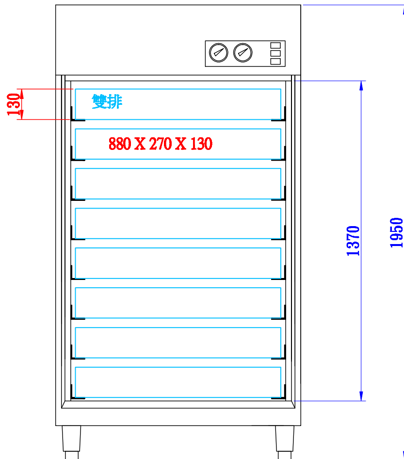
前視圖
