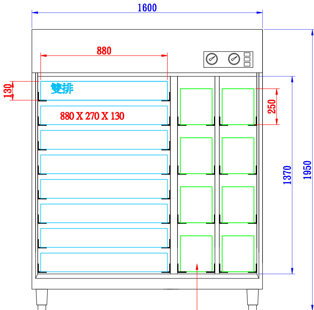
前視圖
