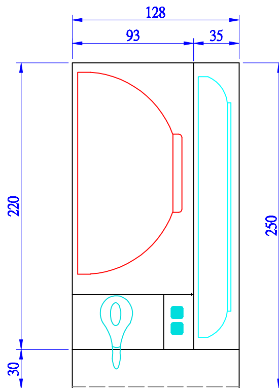
俯視圖
