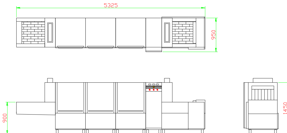
機器外尺寸:
