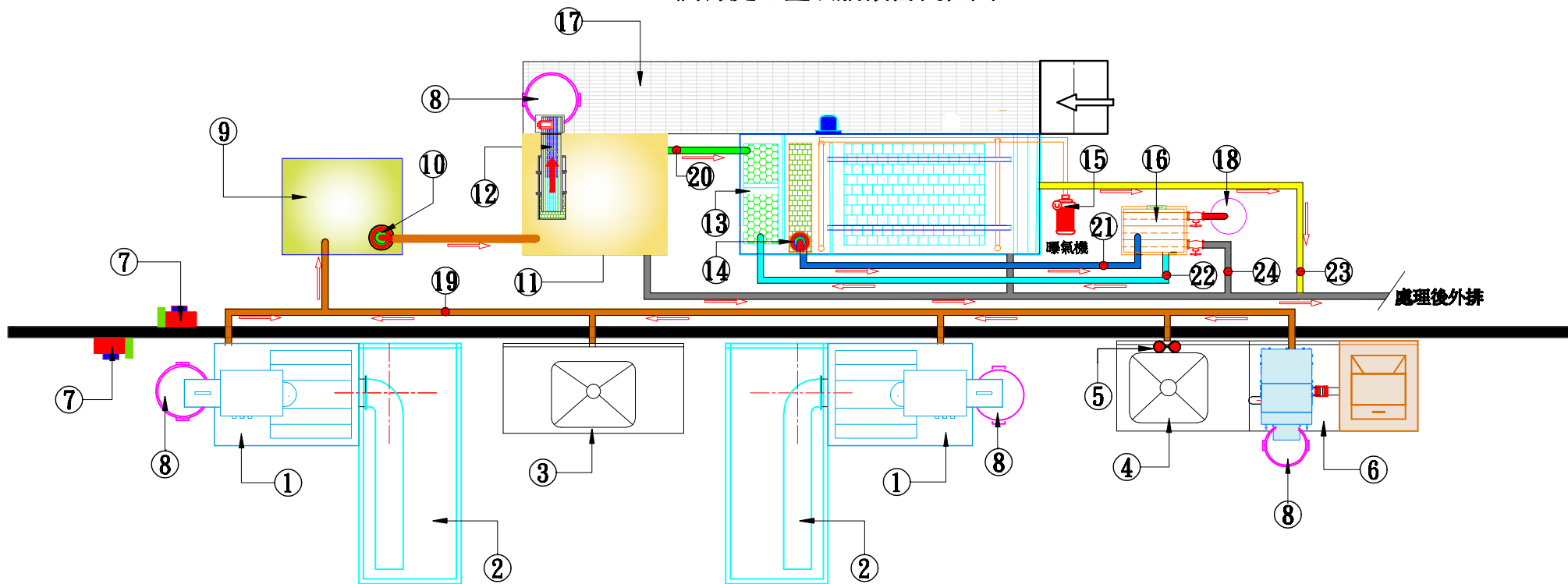
廚餘處理暨油脂截留流程圖
